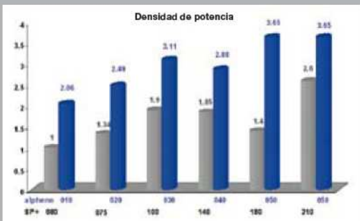
Comparativa de densidad de potencia: estándar industrial con alpheno®
