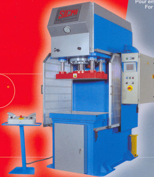
MCL PRESSA VELOCE PER STAMPAGGIO A FREDDO Press for cold pressworks Presse pour emboutissage à froid
